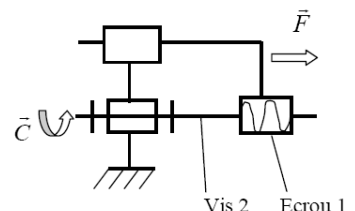
Vis à 2 filets
