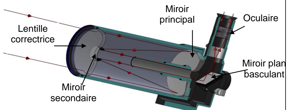
Vue en coupe de l'optique de l'ETX
