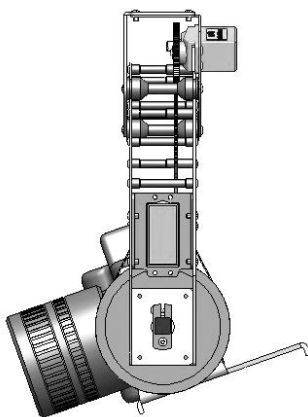
Figure 9 : rotation du plateau
