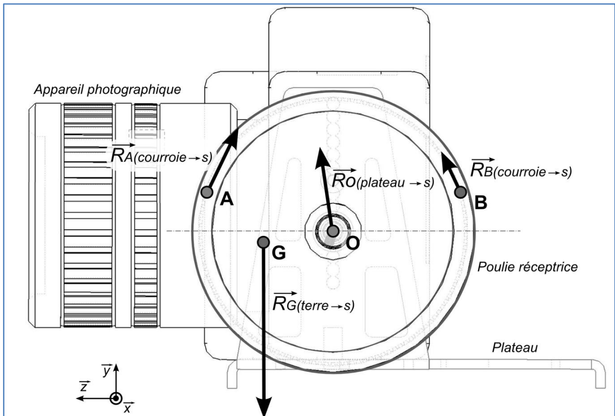
Figure 10 : inventaire des actions mécaniques
