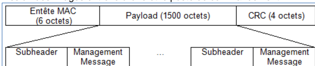
Trame Wimax
